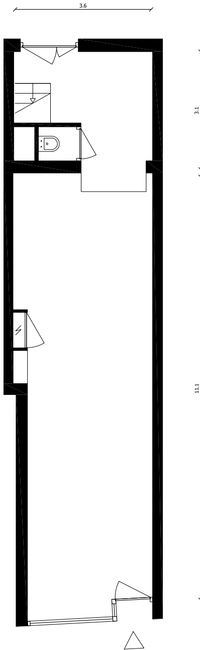
begane grond VVO: 50,1 m 2 BVO: 57,8 m 2
